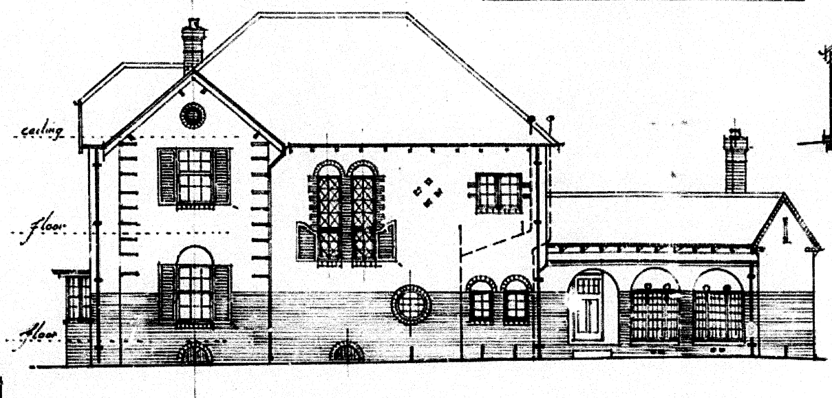
: Elevation to Mentone Rd :
