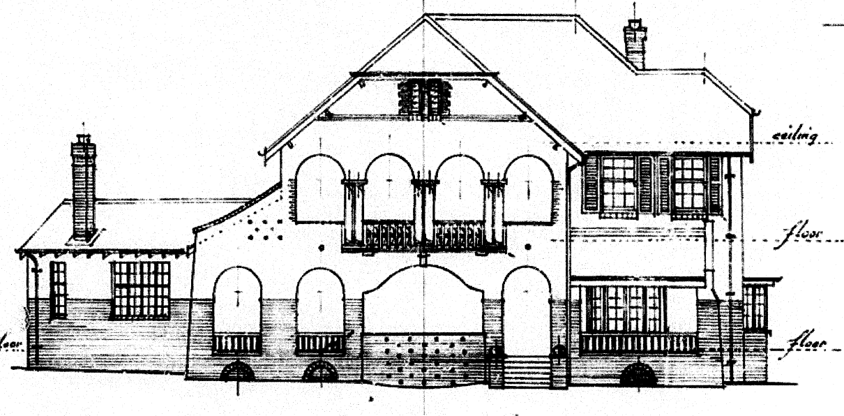
: Elevation facing SE :
