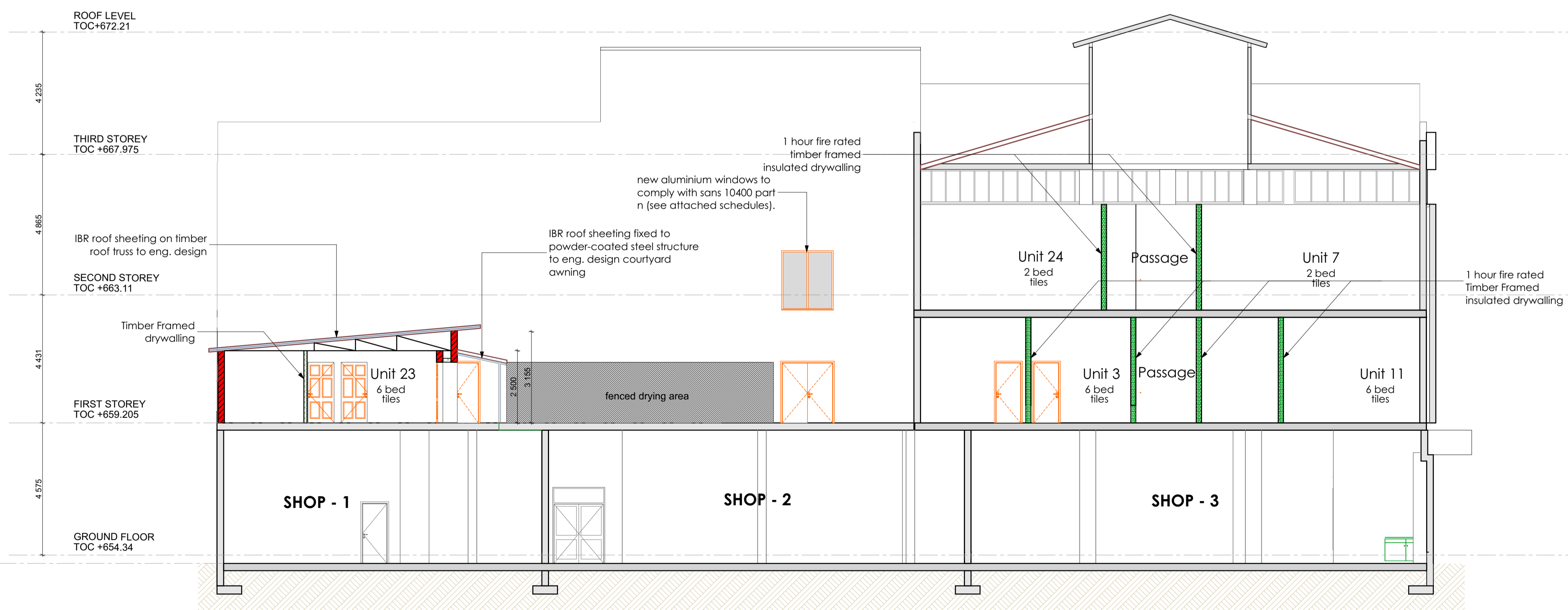
SECTION A-A 1:100
