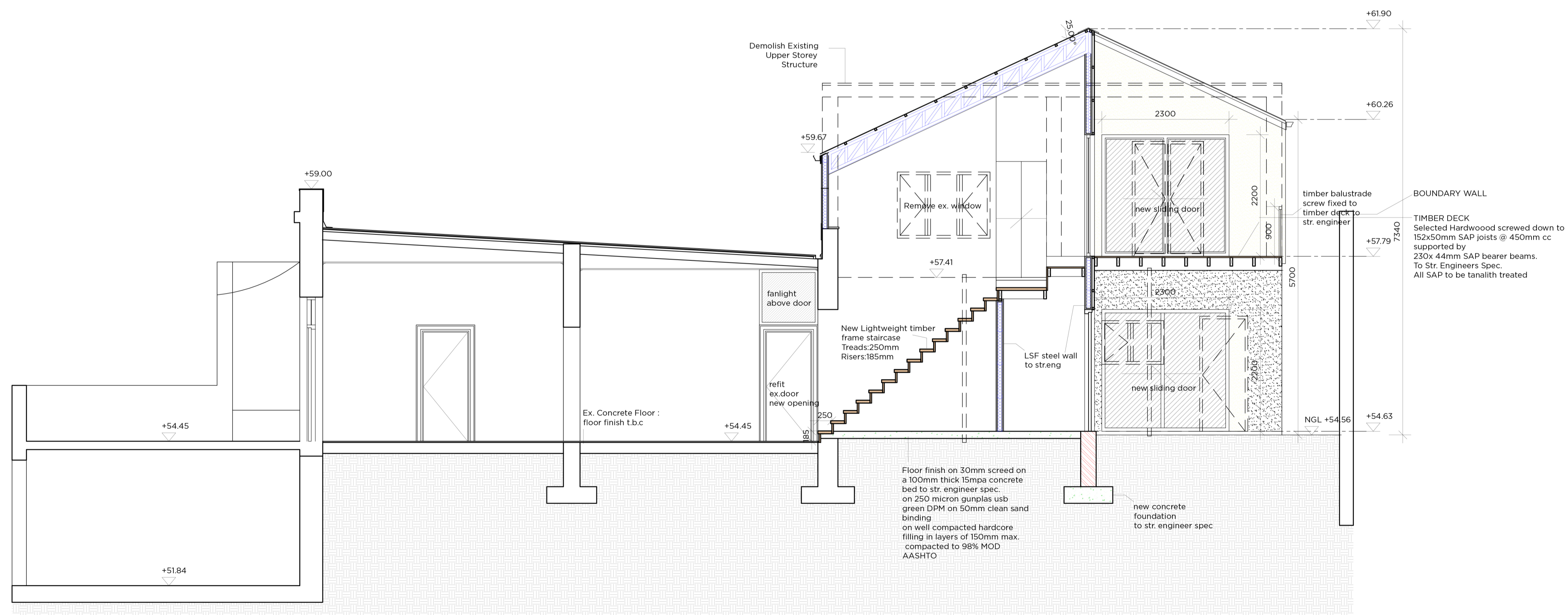
SECTION BB 1:50
