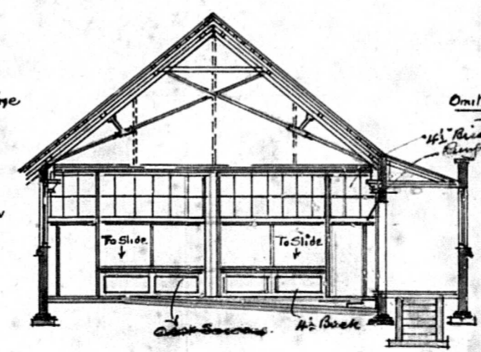
SECTION A-B
