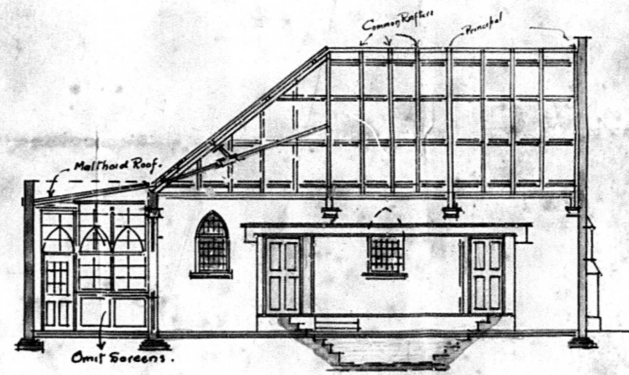
SECTION C-D
