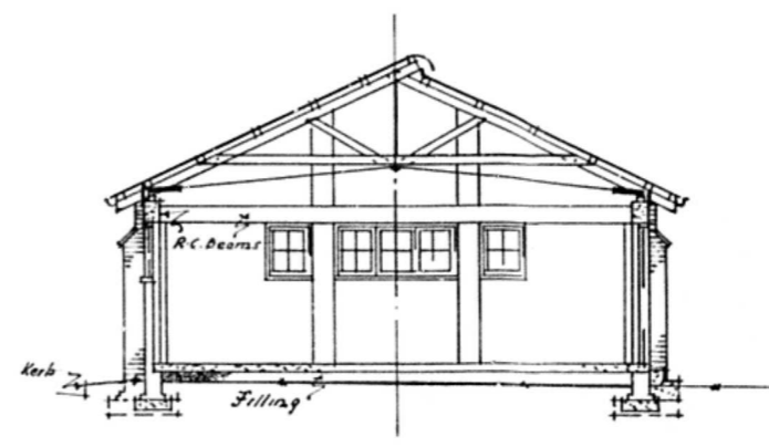
SECTION A-B
