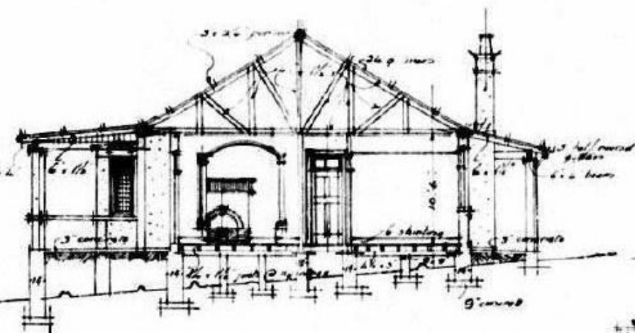
SECTION A-D
