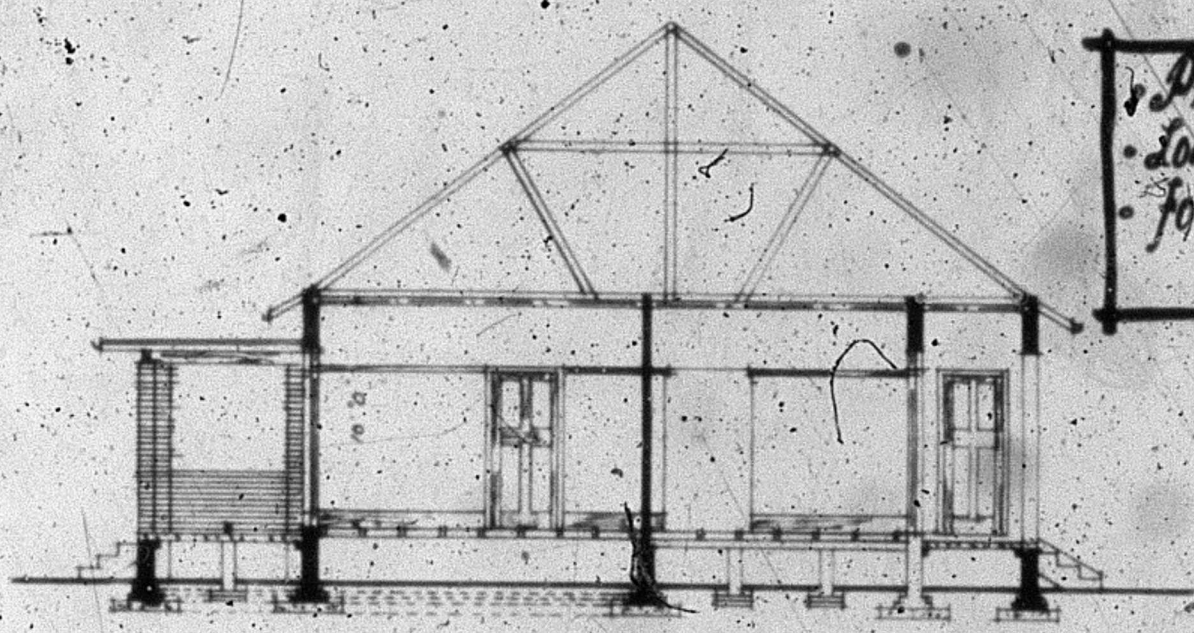
Section A-B
