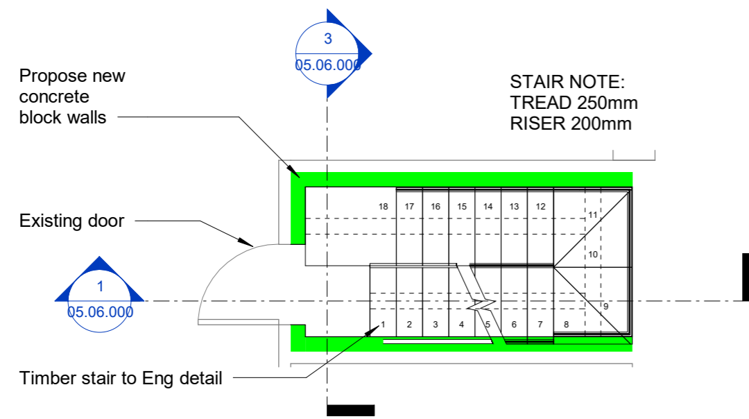
2 STAIR CALLOUT 01.12.000 1 : 50
