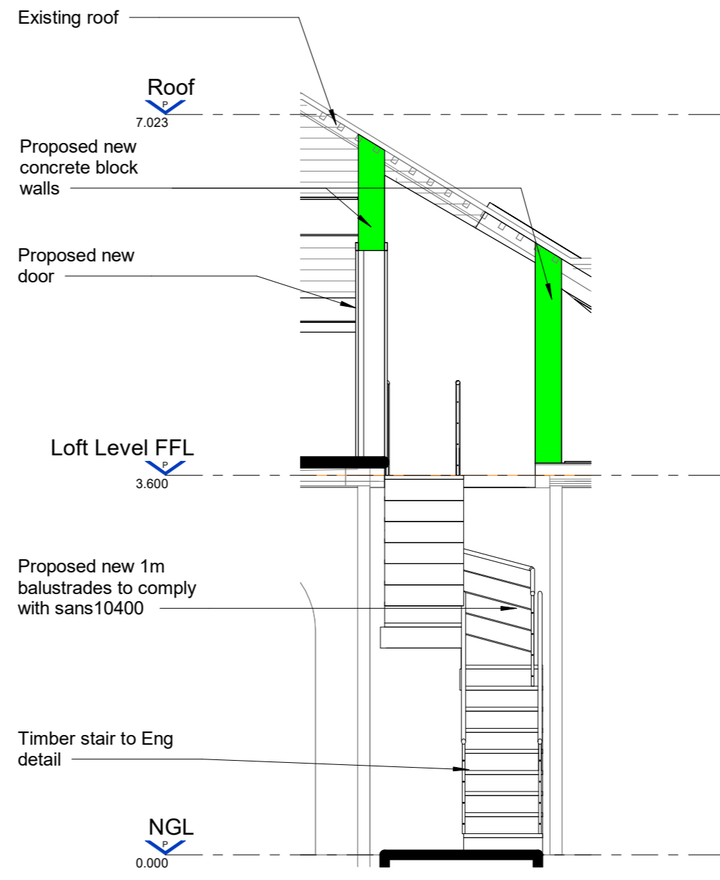
3 STAIR SECTION 02 01.12.000 1 : 50
