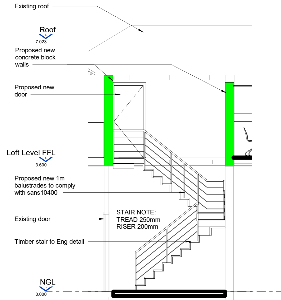
1 STAIR SECTION 01 01.12.000 1 : 50
