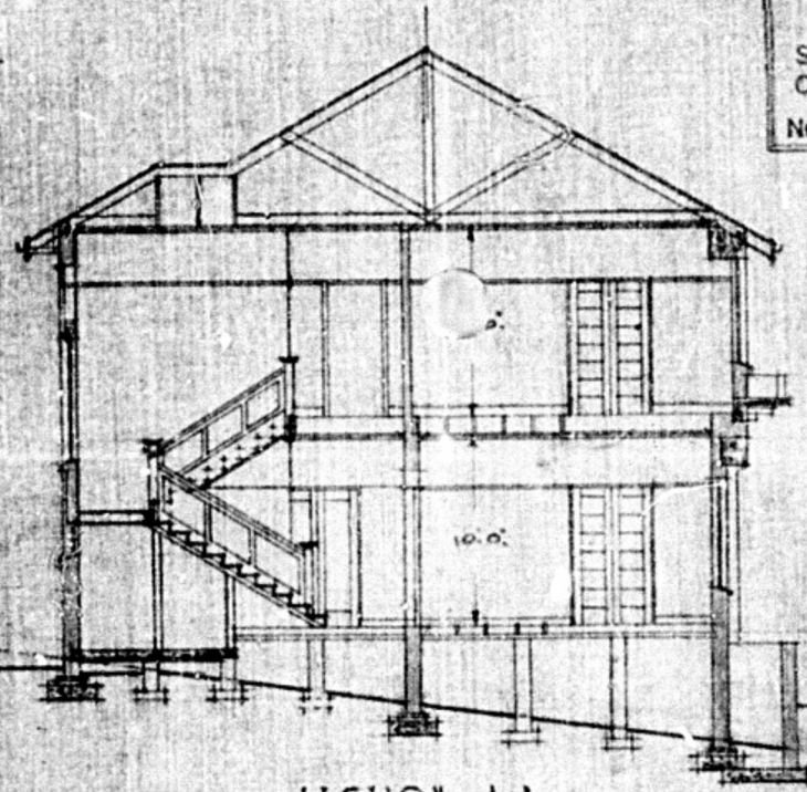
SECTION A-B
