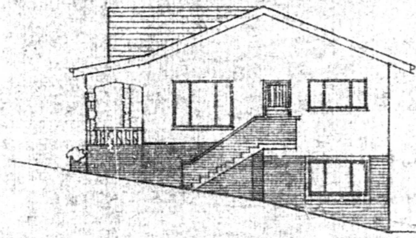
SIDE ELEV.
