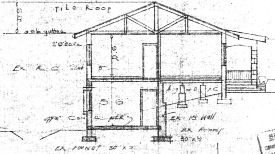
SECTION A-B
