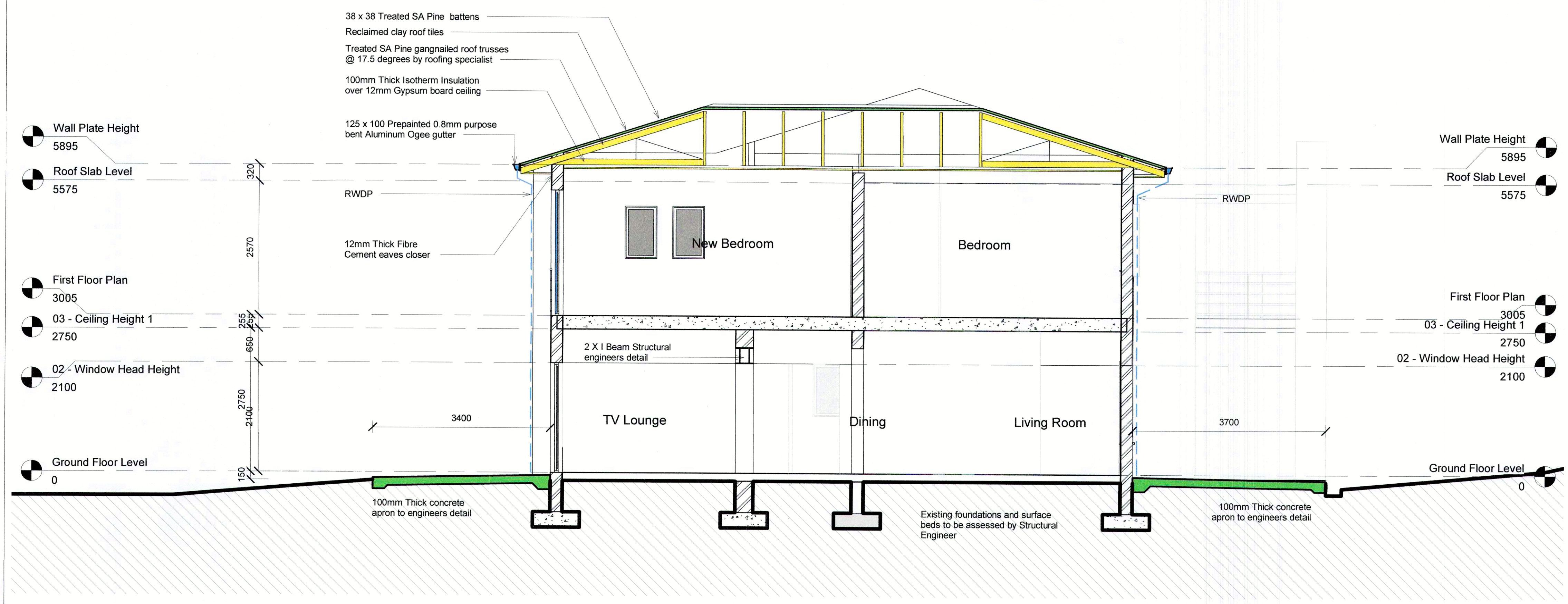
1 Section 1 1 : 50
