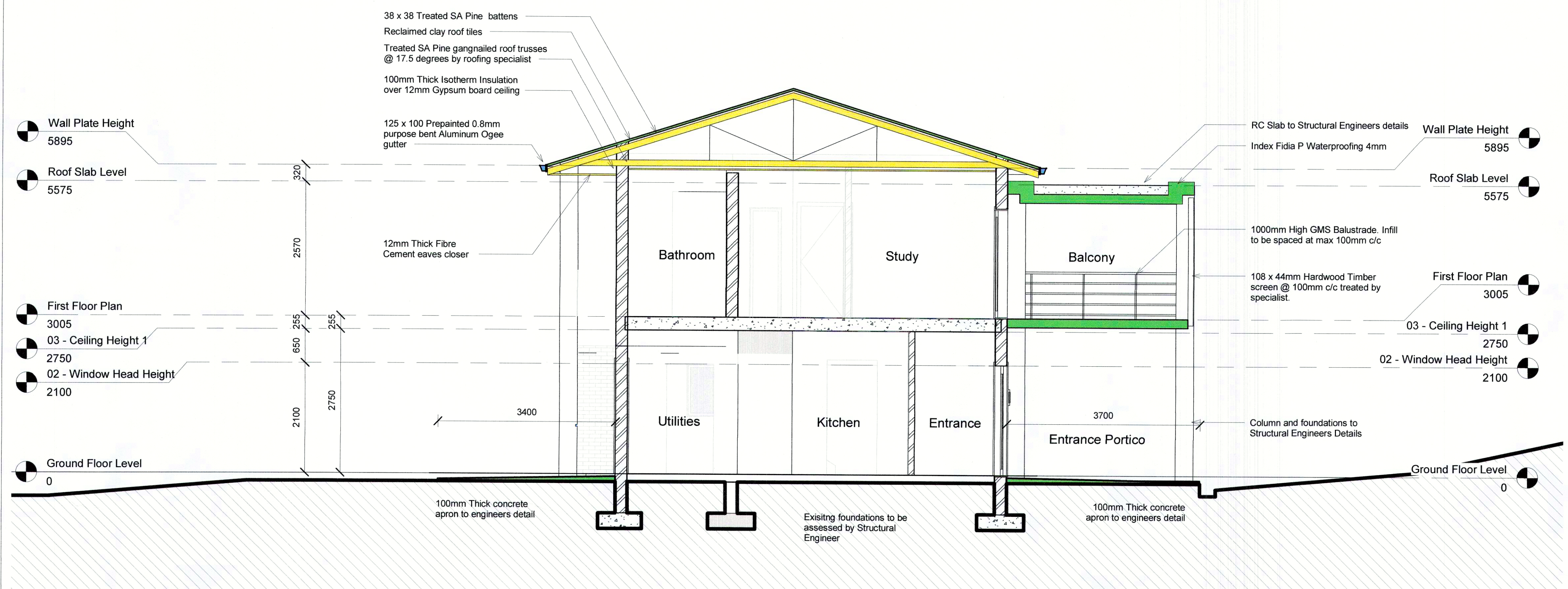
2 Section 2 1 : 50
