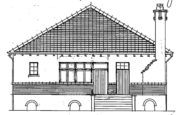
~ BACK ELEVATION ~
