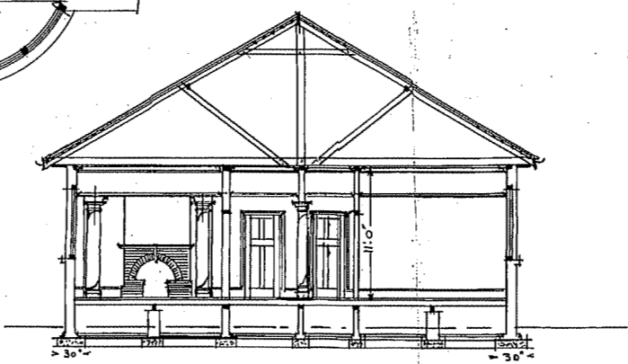
~ SECTION A-B ~
