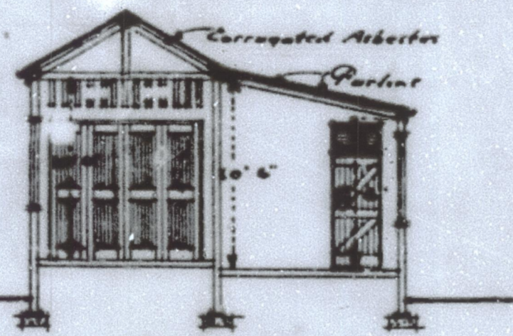
Section A-B
