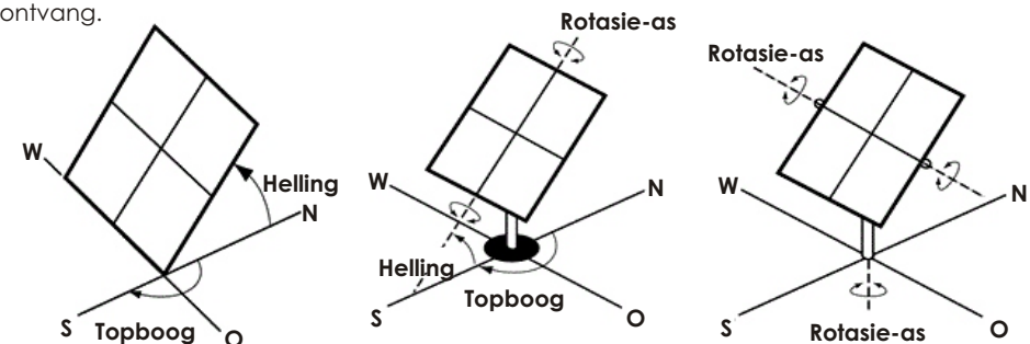
Figuur 3: Oorsig van verskillende FV-naspoorstelsels (van links na regs: vastehoek-, enkelasnasporing en dubbelasnasporing (bron: pveducation.com)).
