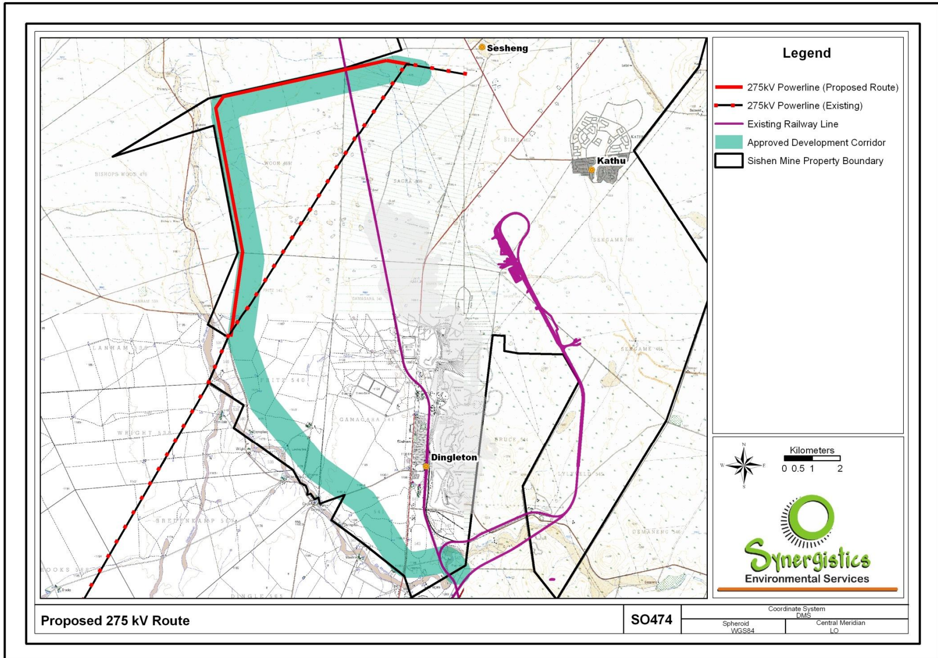
Figuur 1: Ligging van die bestaande en voorgestelde roete vir die ~12 km gedeelte van die 275 kV kraglyn wat hervestig moet word.
