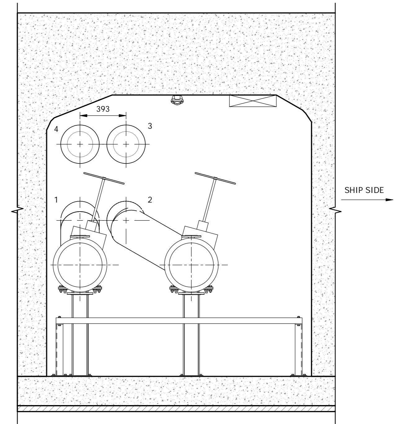
SECTION B - B 1 : 20
