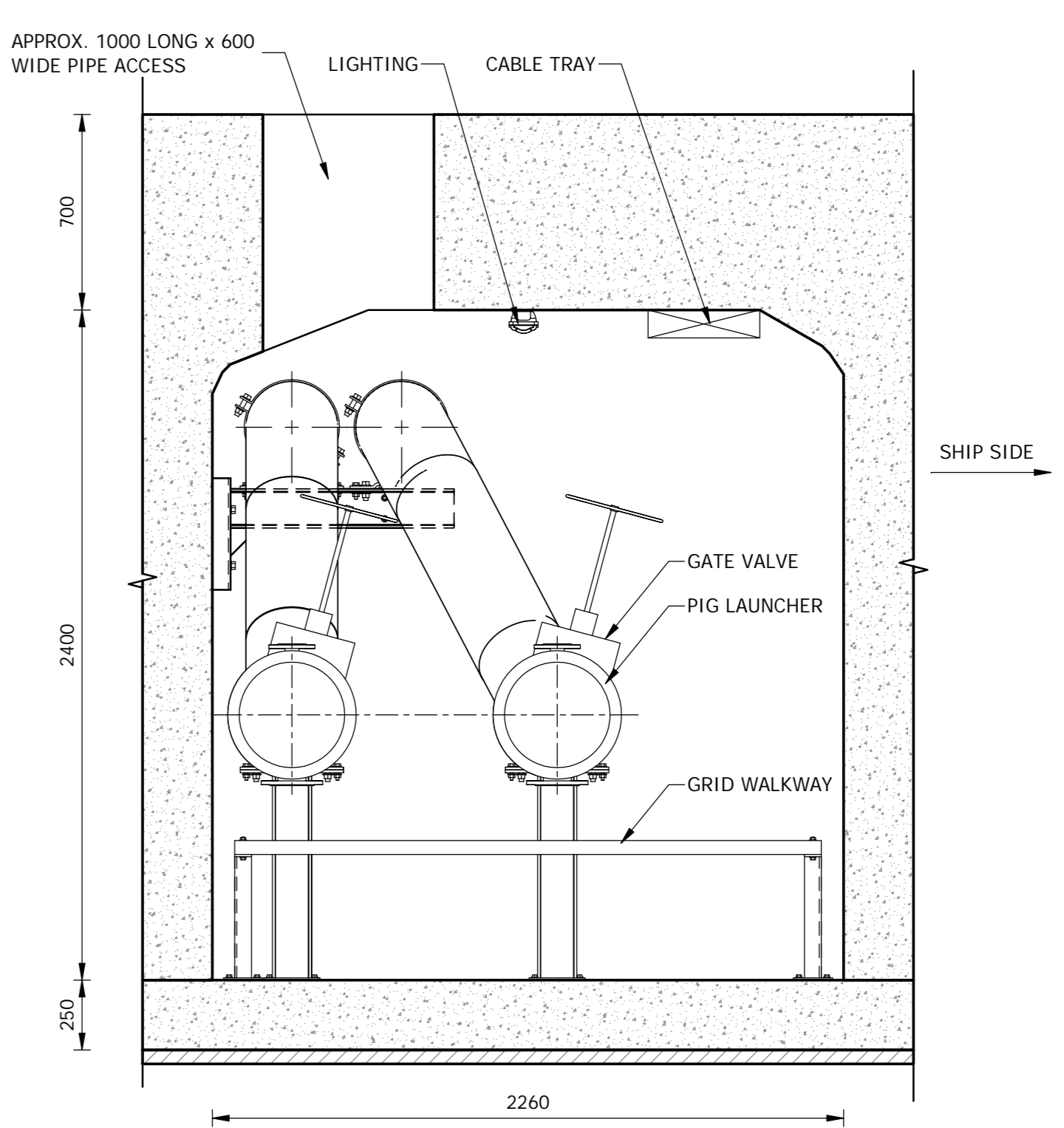
SECTION A - A 1 : 20
