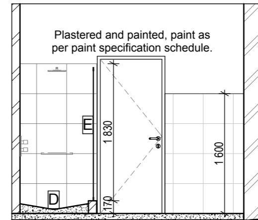
1 ELEVATION 1 1:50
