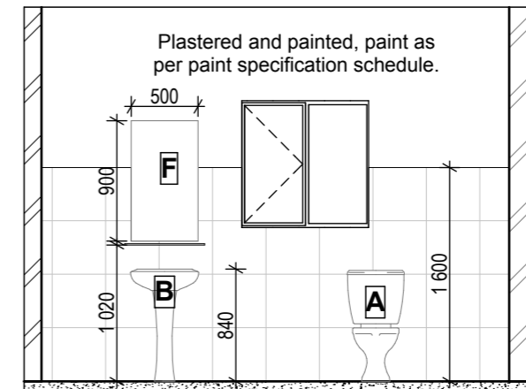
2 ELEVATION 2 1:50
