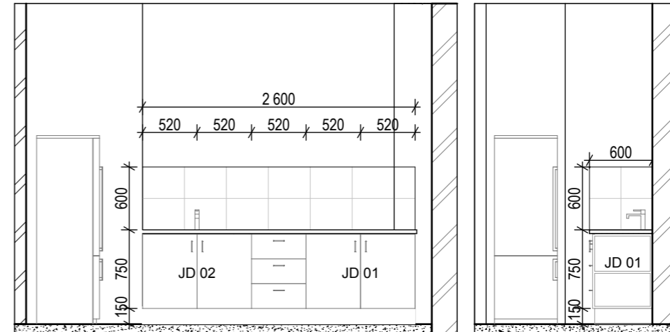
1 ELEVATION R1 1:50 2 SECTION R1 1:50
