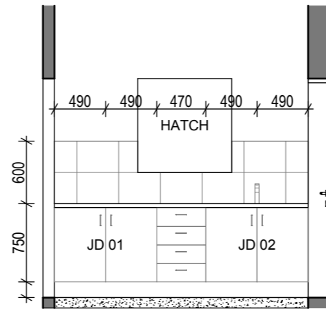
3 ELEVATION B 1:50
