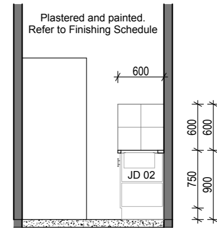
4 ELEVATION C 1:50
