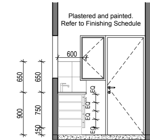
2 ELEVATION A 1:50
