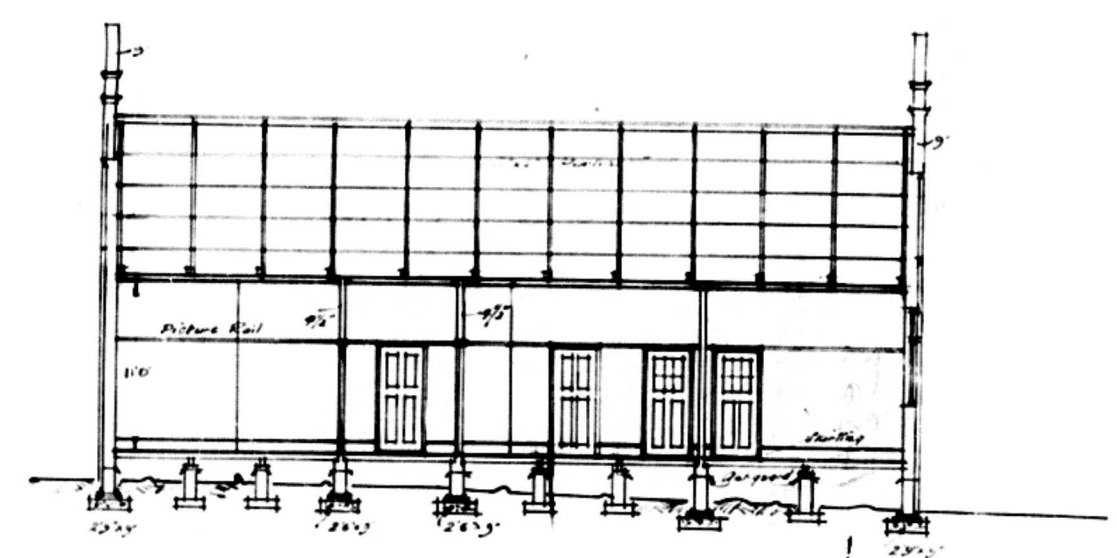
Section A-B.
