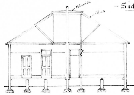
— Section A B C D —
