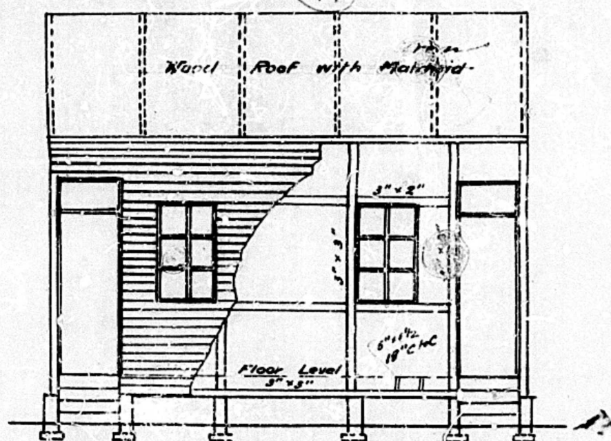
Elevation
