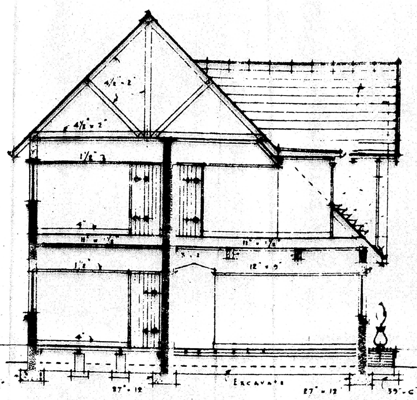
SECTION A-D
