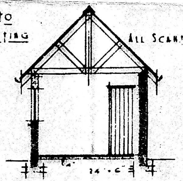
SECTION C-D
