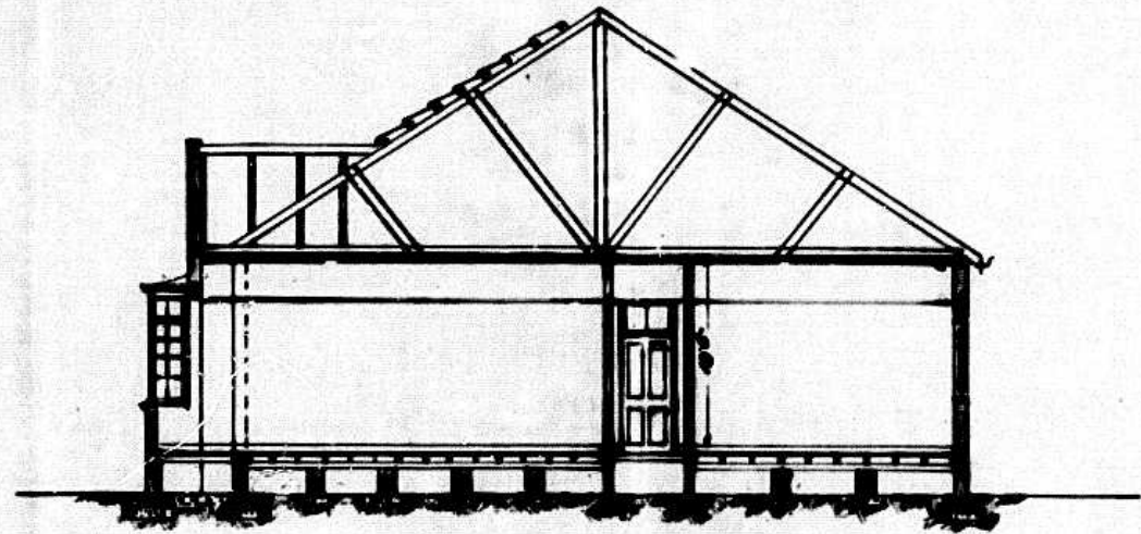
— SECTION A.B. —
