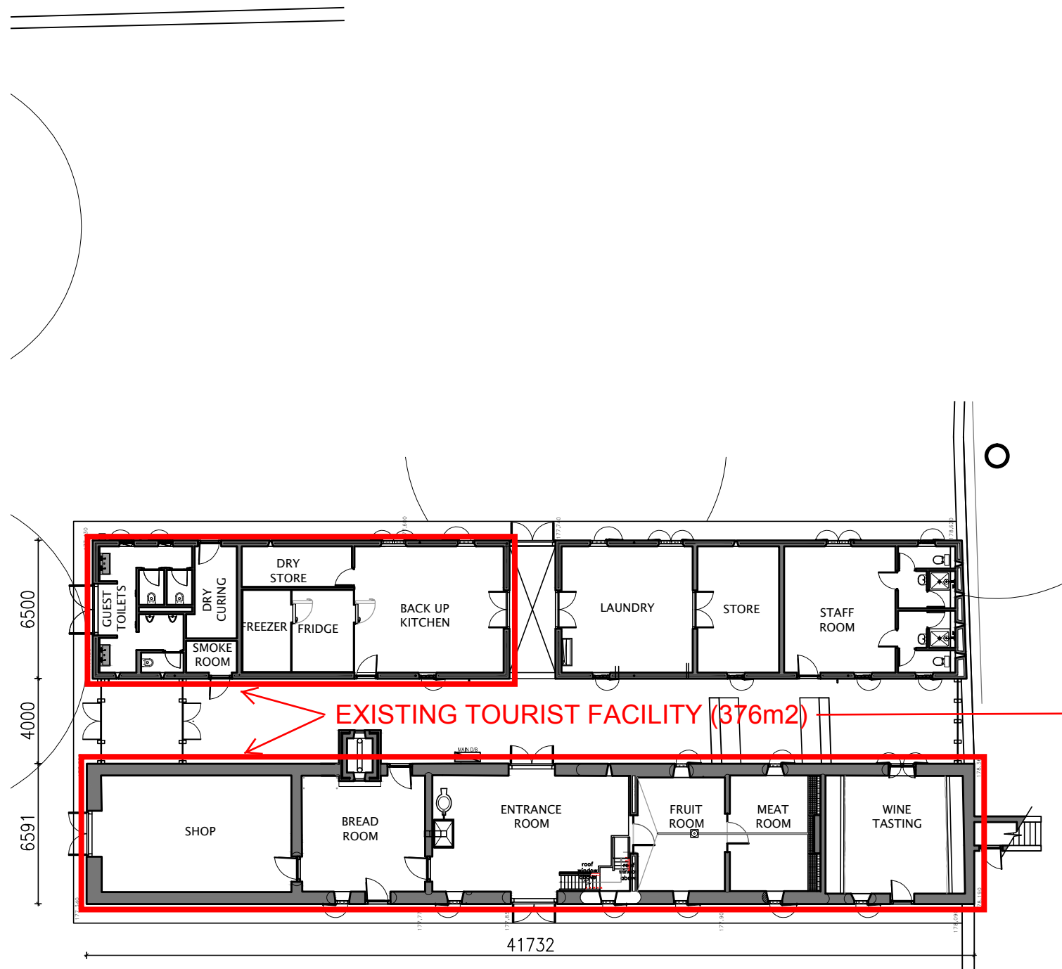
EXISTING FLOOR PLAN 1:250 @A3 5 TOILETS
