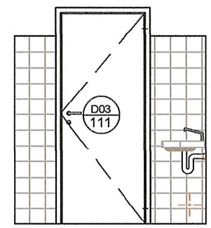
Elevation 3 - a
