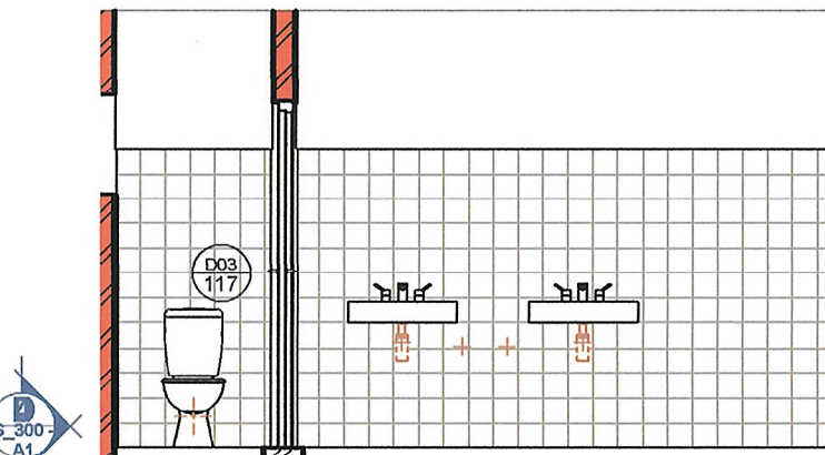
Elevation 2 - b
