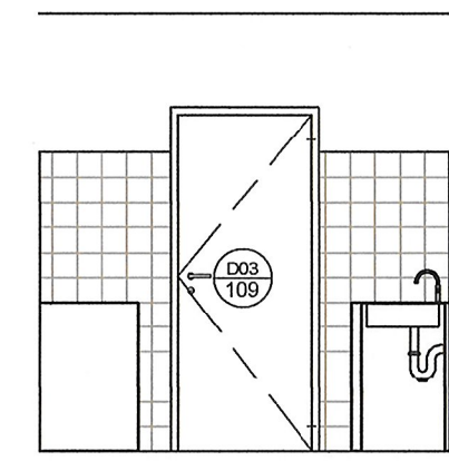
Elevation 1 - d
