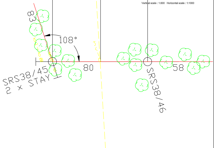
Vertical scale : 1:500 Horizontal scale : 1:1000
