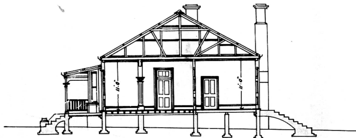
Section AB.
