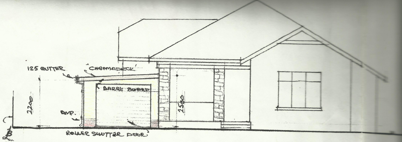
S.E. ELEVATION
