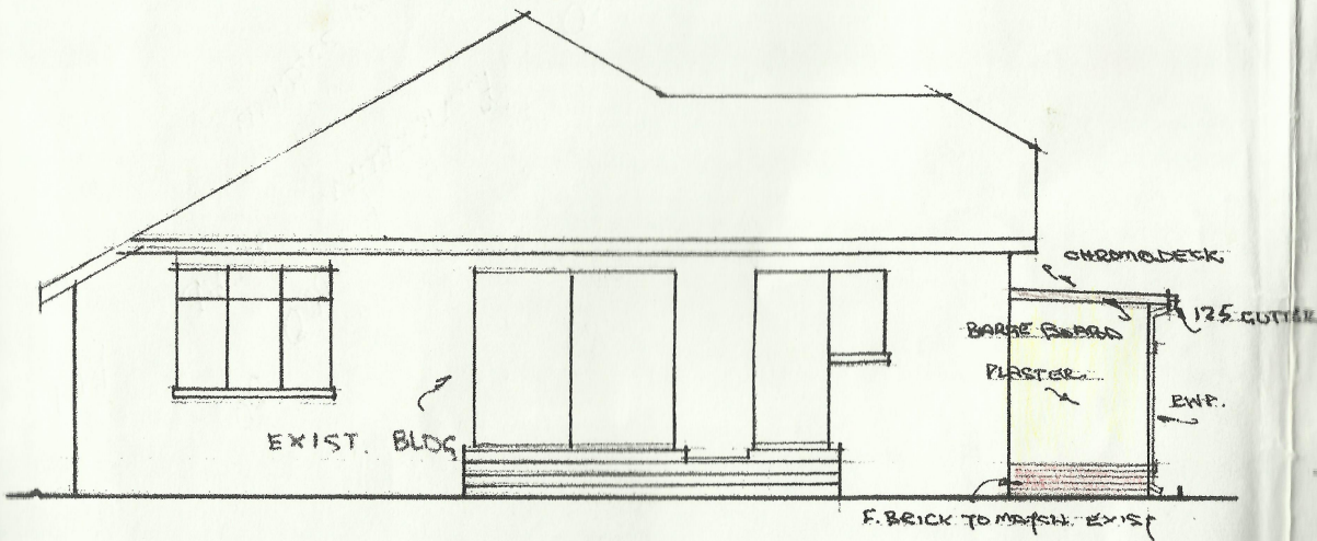
N.W. ELEVATION
