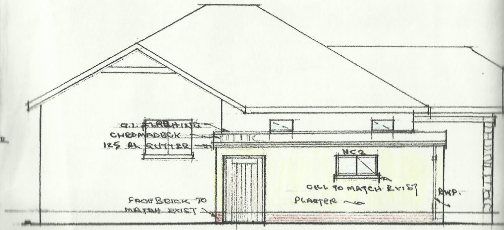
S.W. ELEVATION
