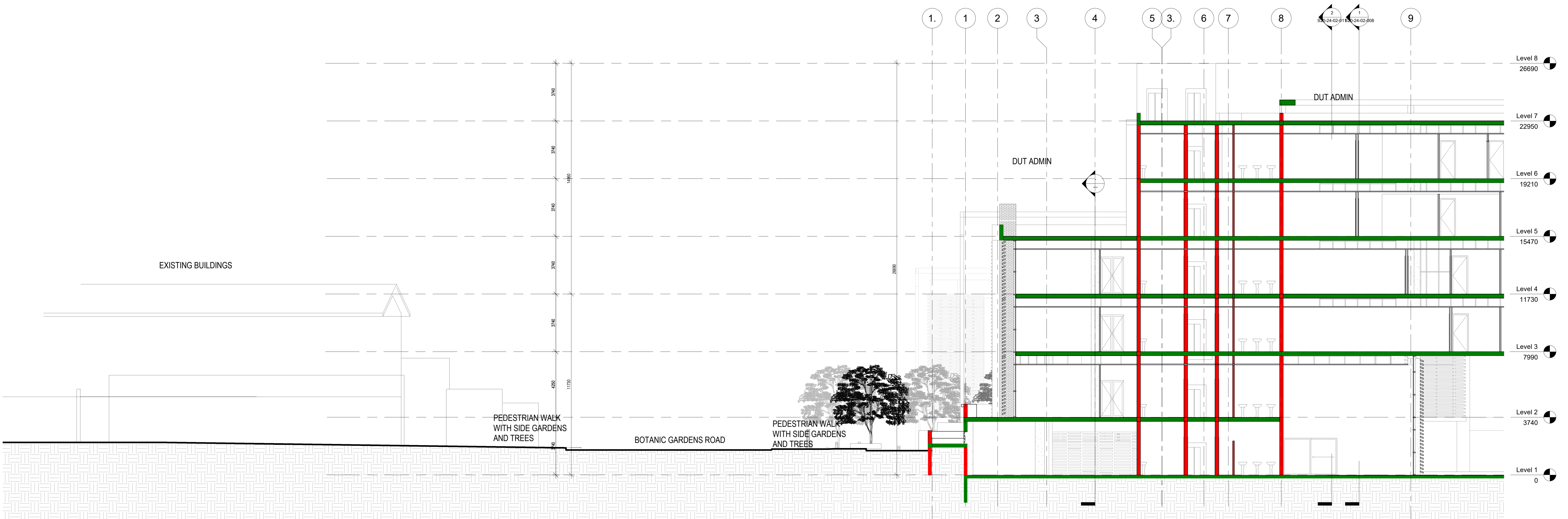
1 SITE CONTEXT SECTION 6 1 : 100
