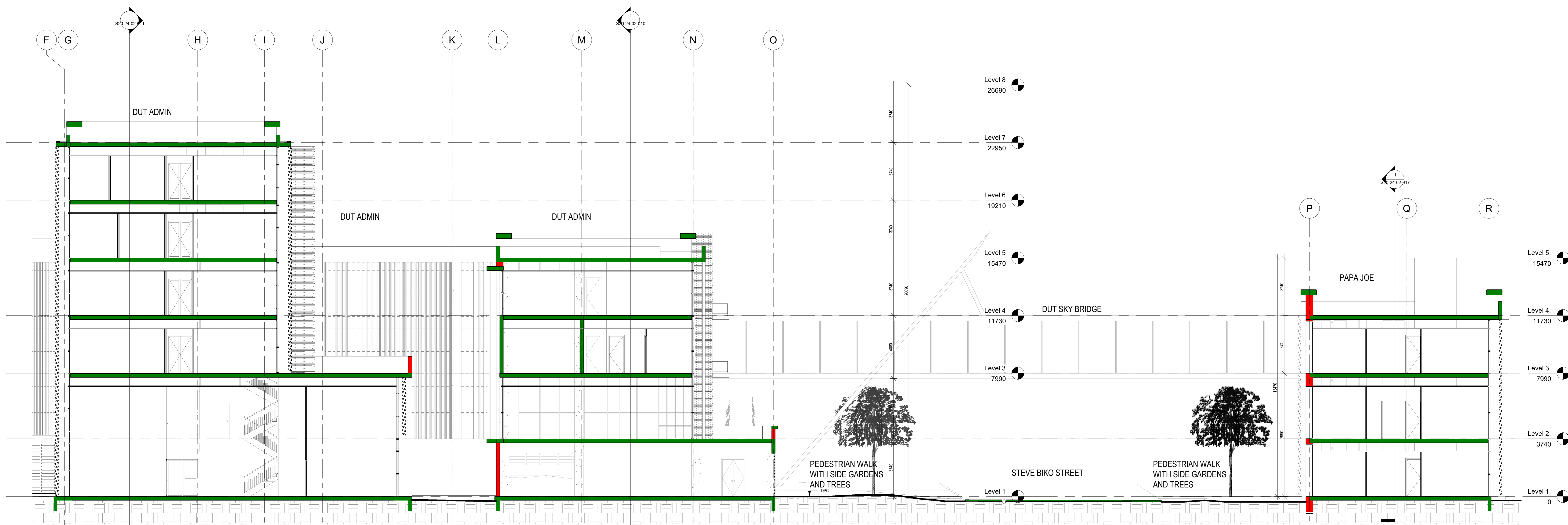
2 SITE CONTEXT SECTION 5 1 : 100
