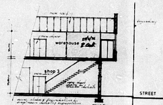
section D-D 1:100
