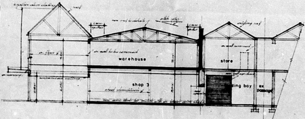
section A-A scale 1:100
