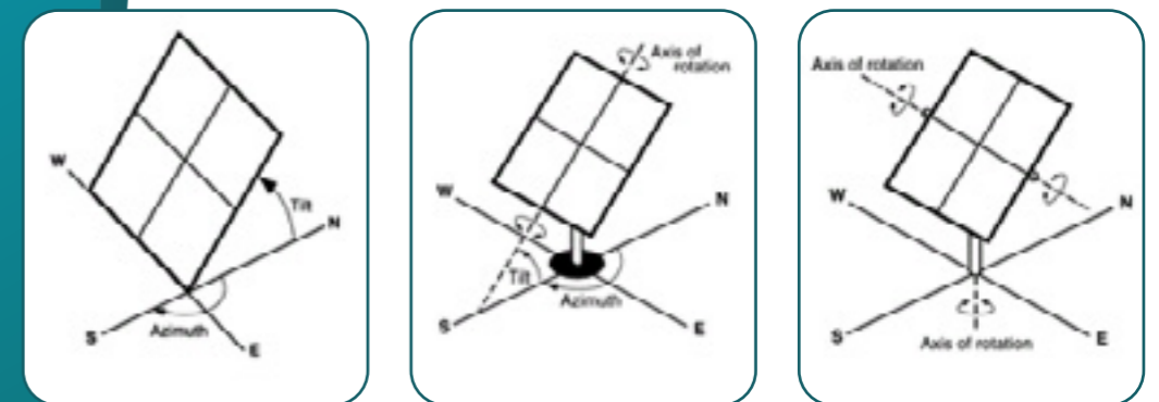
Figuur 3: Oorsig van verskillende FV-naspoorstelsels (van links na regs: vastehoek, enkel- en dubbelaspooring (bron: pveducation.com))
