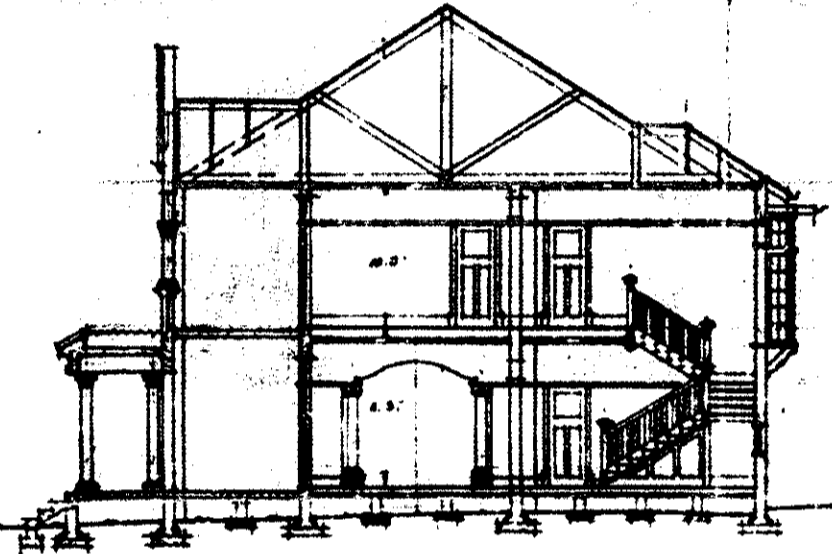
SECTION A-B
