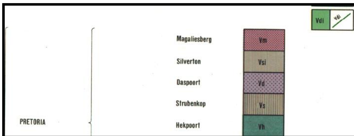
Figure 4: Lithostratigraphy (Walraven 1978).
