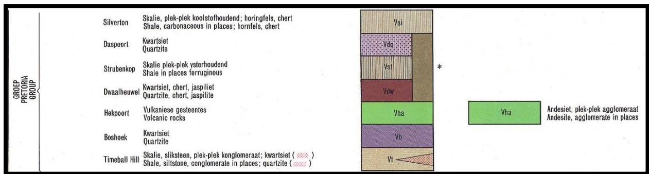
Figure 4: Lithostratigraphy (Walraven 1978).
