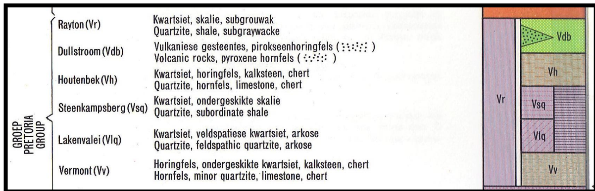
Figure 4: Lithostratigraphy (Walraven 1978).
